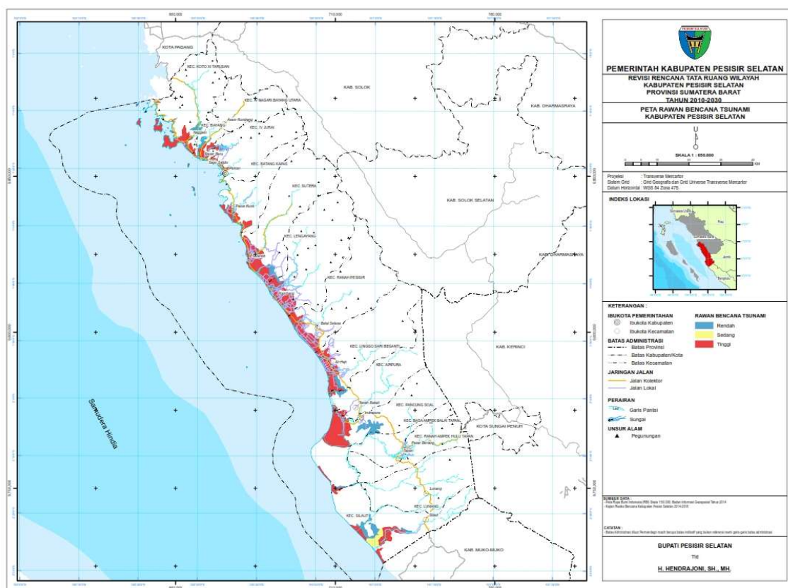
Gambar 2.18 Peta Rawan Bencana Tsunami
